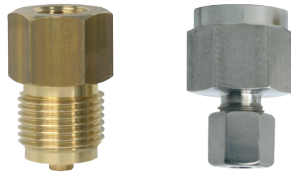
Fig. izq.: Racores macho-hembra, G ½ / G ¼ B
