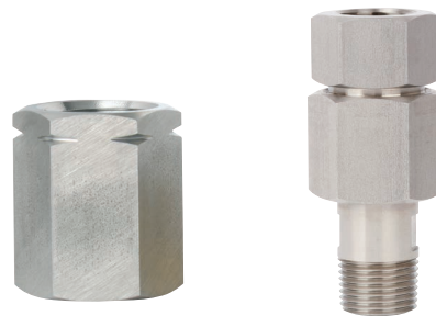
Fig. izq.: Racor, manguito de sujeción, rosca ½ / rosca ¼ B
