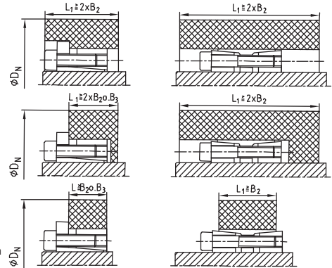
Condiciones montaje elto. de fijación
