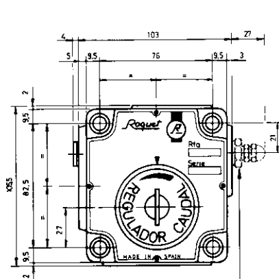
Situación válvula limitadora (opcional) Optional relief valve position
