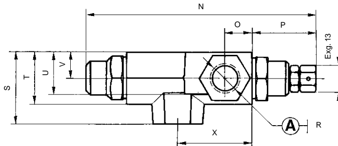
▲ Regulación forma 2 Adjusting type
