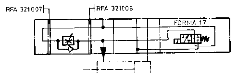
VARIANTE 1: Regulación por "A" en la salida. Velocidad rápida. VERSION1: Fast meter in.
