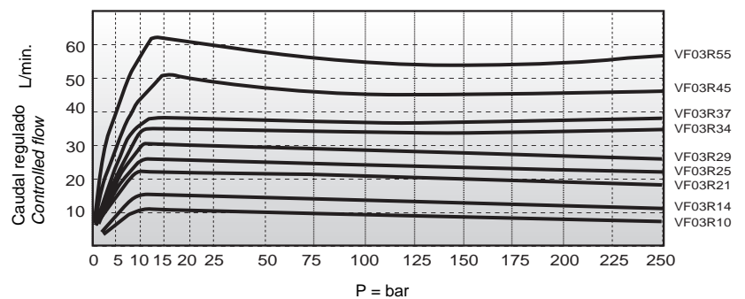
DIAGRAMA: Presión-caudal DIAGRAM: Pressure-flow rate A→B
