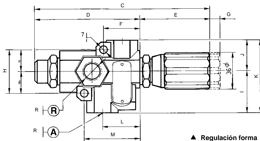
▲ Regulación forma 3 Adjusting type 3
