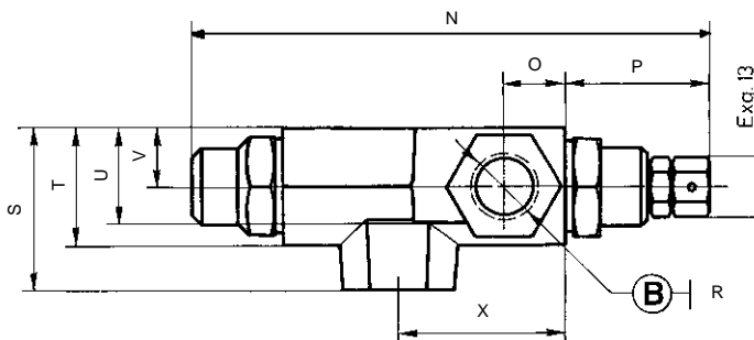
▲ Regulación forma 2 Adjusting type 2
