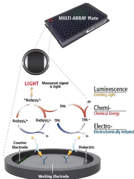
Figura 9. Esquema de funcionamiento de un ECLIA
