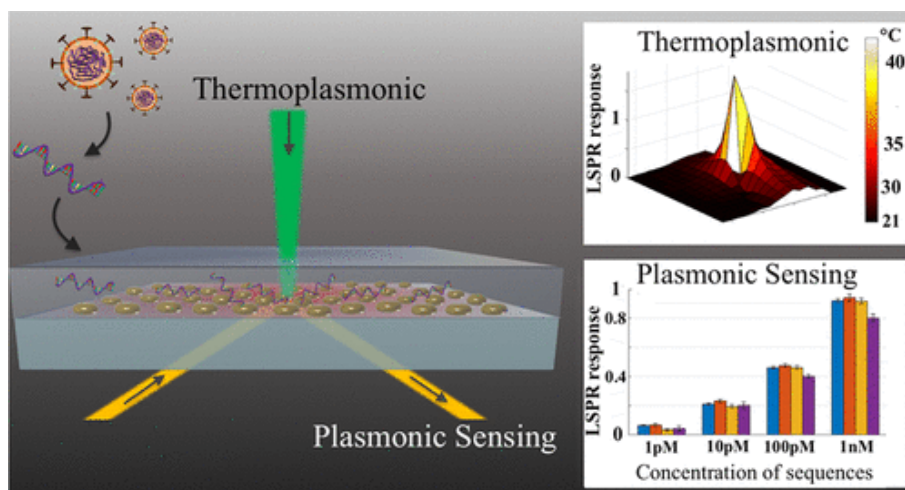
Figura 19. Esquema del principio de funcionamiento del biosensor plasmónico y la respuesta obtenida en el rango de 1-1000 pM de oligonucleótidos específicos de COVID-19
