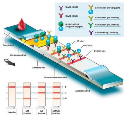
Figura 8. Esquema del funcionamiento de un test serológico en formato LFIA (253)
