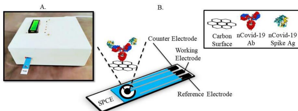
Figura 26. A. Diseño de la plataforma de biosensado eCovSens. B. Esquema de funcionalización de los electrodos serigrafados con los anticuerpos monoclonales, seguido de la adición de la muestra que contiene
