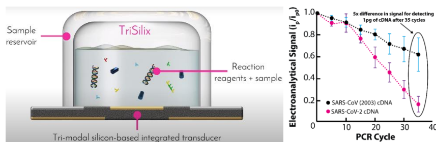
Figura 21. Diseño del chip de silicio "TriSilix" en que se puede realizar los procesos de amplificación, medición de temperatura y detección electroquímica de oligonucleótidos de COVID-19 usando azul de metileno como sonda redox. A medida que se repiten los ciclos de replicación la señal electroquímica del azul de metileno disminuye por su interacción con las cadenas de cDNA viral.
