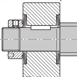
Sujeción con muelle de plato
