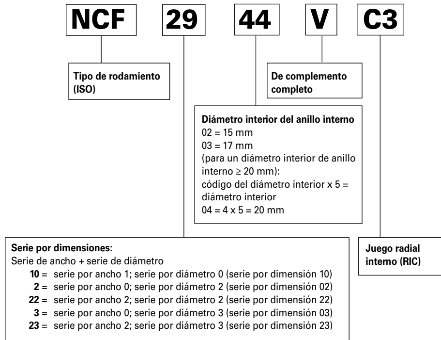
Fig. 20. Nomenclatura para rodamiento de rodillos cilíndricos full-complement (NCF).
