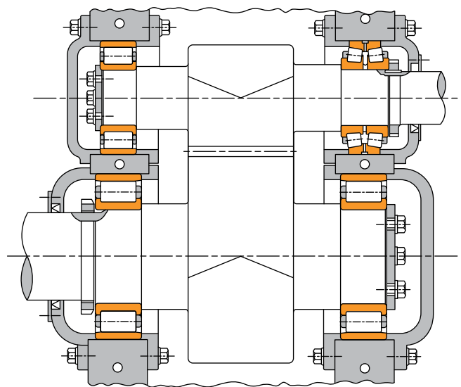
Fig. 11. Caja reductora de reducción simple.
