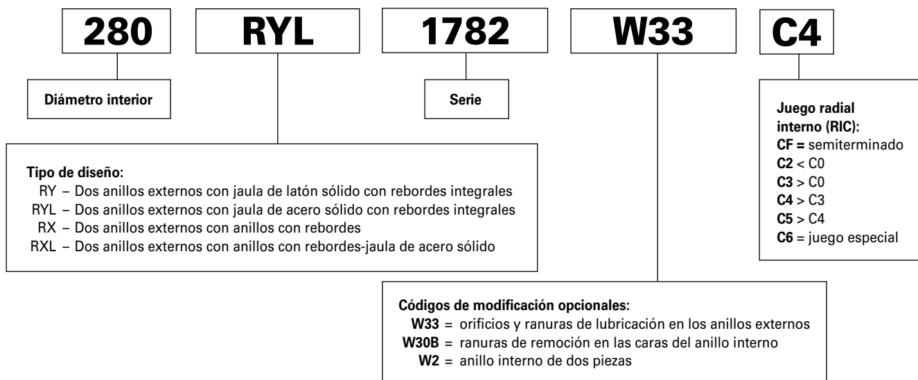
Fig. 38. Nomenclatura del conjunto de rodamientos de rodillos cilíndricos de cuatro hileras.
