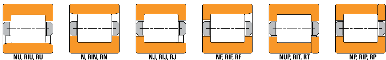
Fig. 1. Rodamientos de rodillos cilíndricos radiales.
