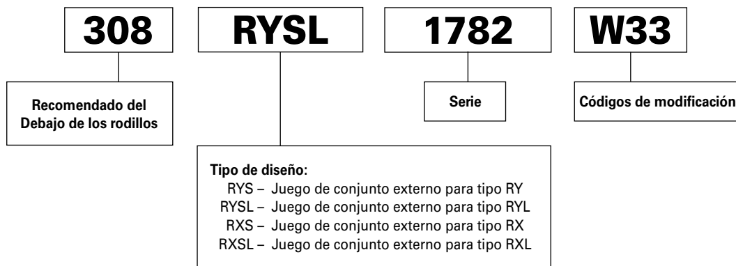
Fig. 40. Nomenclatura del conjunto externo de rodillos cilíndricos de cuatro hileras
