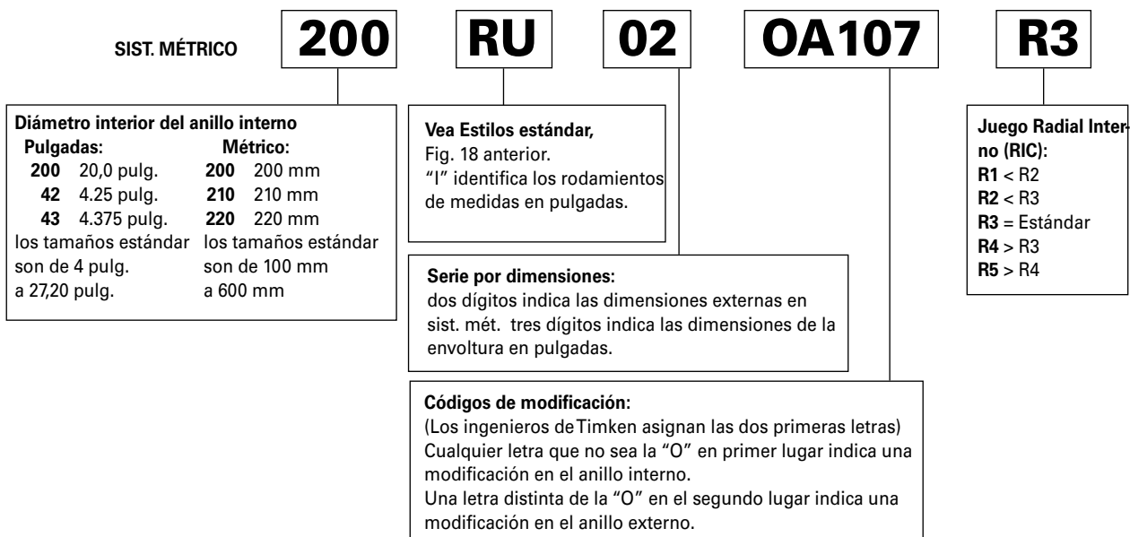
Fig. 19. Nomenclatura de rodamientos de rodillos cilíndricos radiales ABMA.
