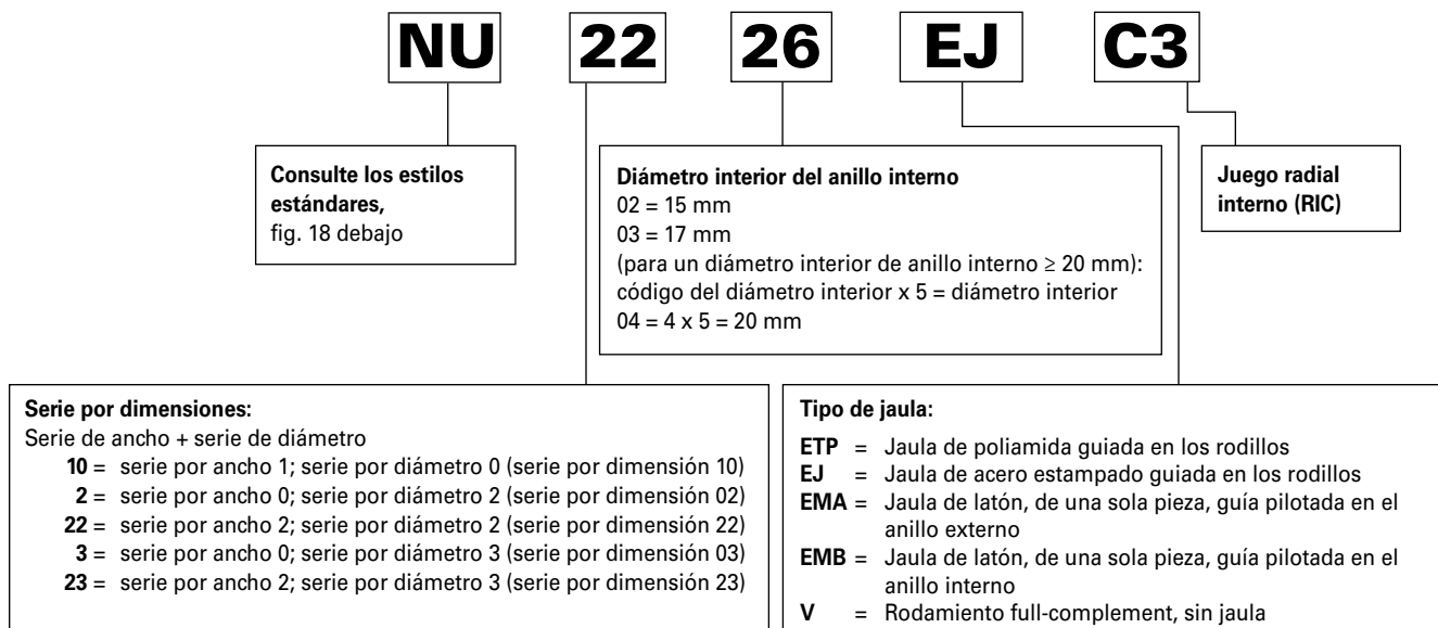
Fig. 17. Nomenclatura de rodamiento de rodillos cilíndricos radiales, sistema métrico ISO.
