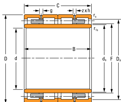
Fig. 23. Rodamiento de rodillos cilíndricos.
