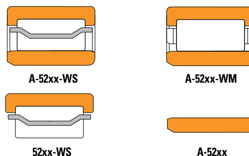
Fig. 2. Rodamientos de la serie de sistema métrico 5200
