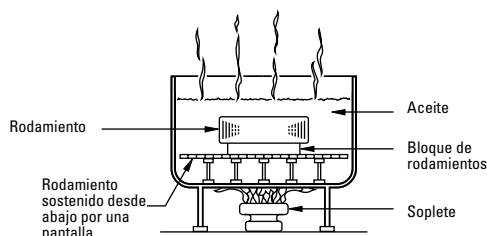
Fig. 12. Método de expansión por calor.
