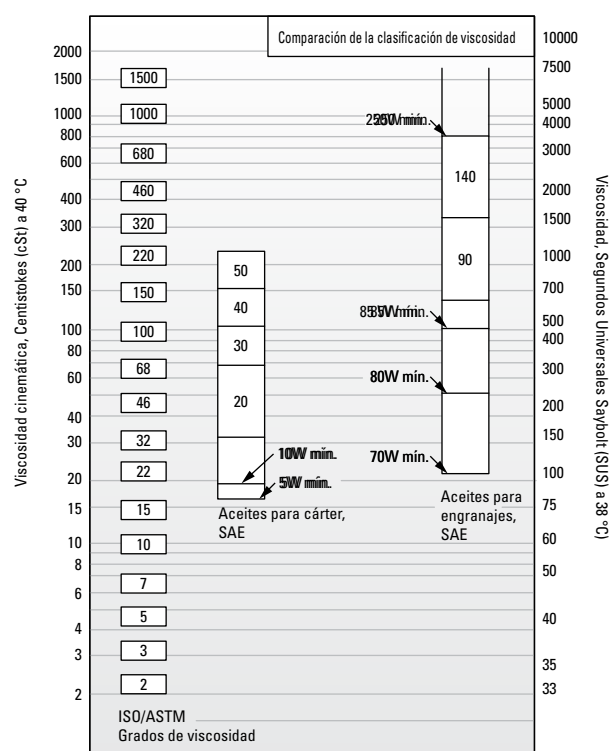
Fig. 13. Comparación entre grados ISO/ASTM (ISO 3448/ASTM D2442) y grados SAE (SAE J 300-80 para aceites de cárter, SAE J 306-81 para aceites de ejes y transmisión manual).
