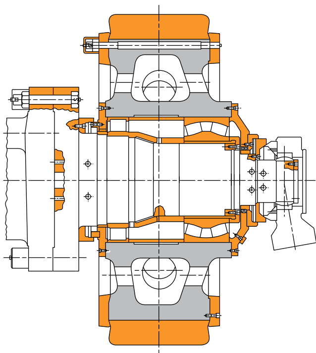
Fig. 10. Conjunto pulverizador de ruedas.
