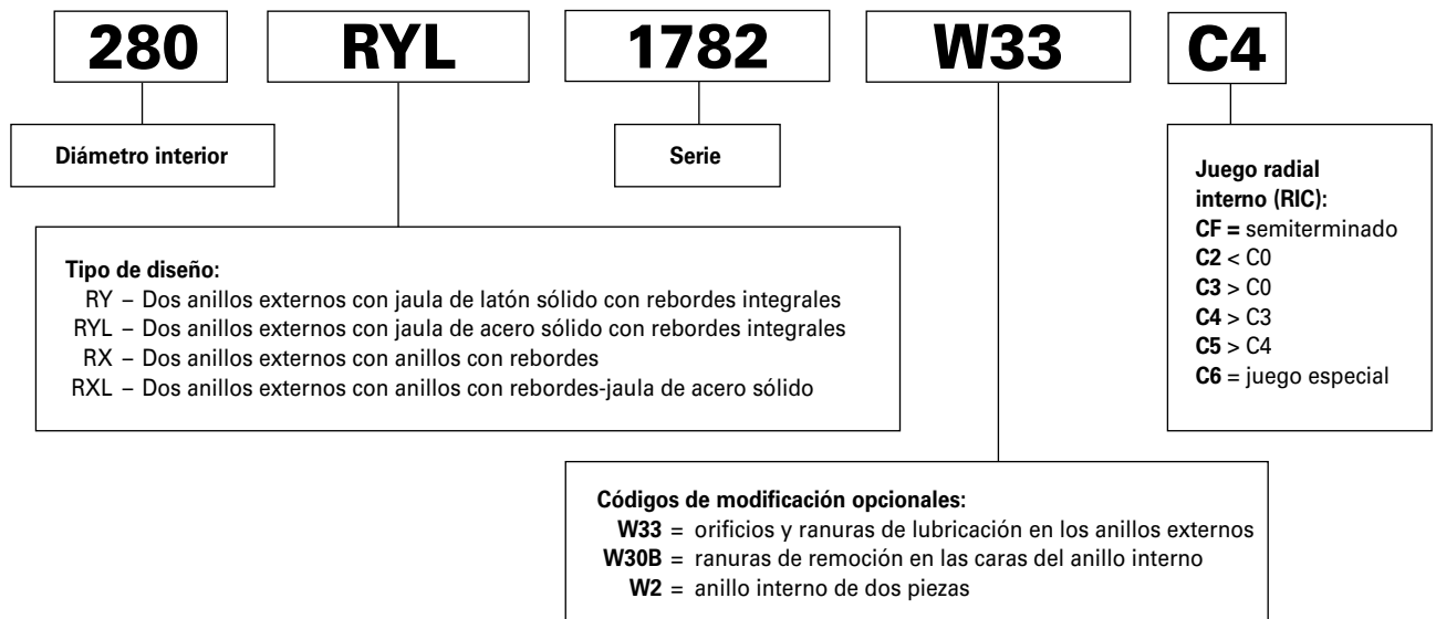
Fig. 21. Nomenclatura de los rodamientos de rodillos cilíndricos de cuatro hileras.
