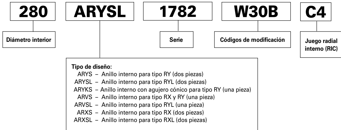
Fig. 39. Nomenclatura de los anillos internos de rodillos cilíndricos de cuatro hileras.
