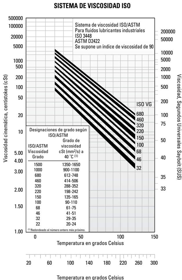
Fig. 14. Sistema de grados de viscosidad para aceites industriales.
